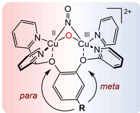
HAT reactivity
